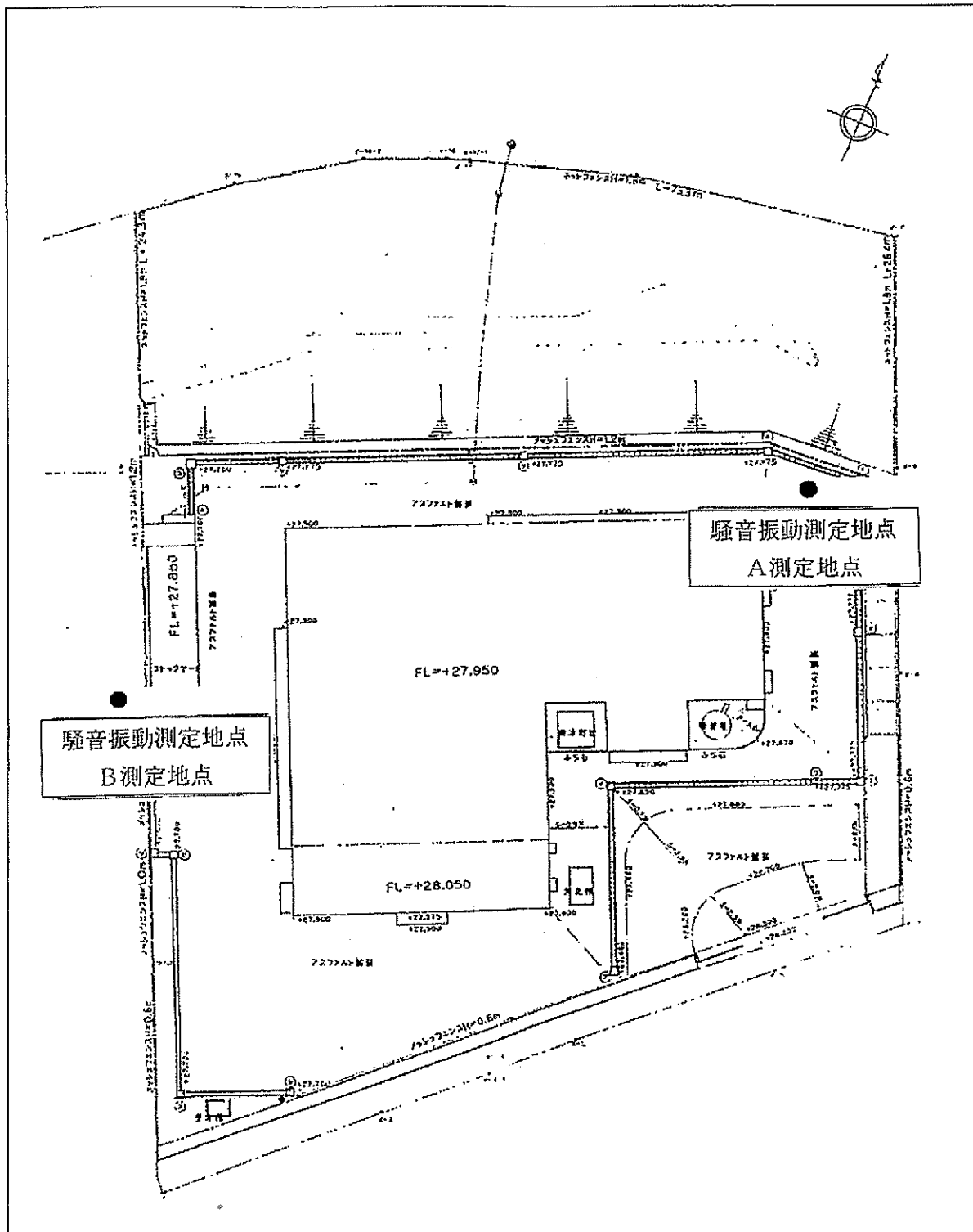
測定点位置図
